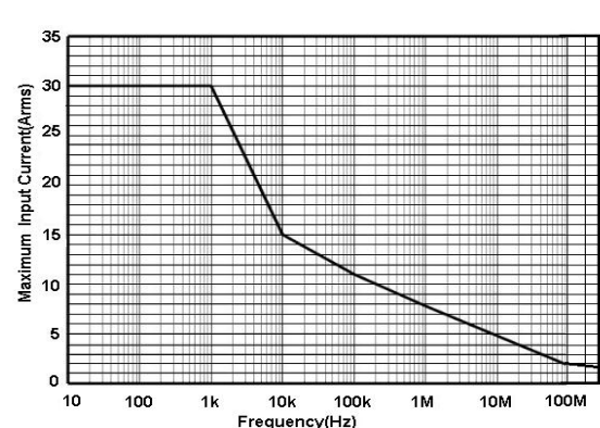
图 2.d HCP8030H 最大测量电流 VS 频率曲线
